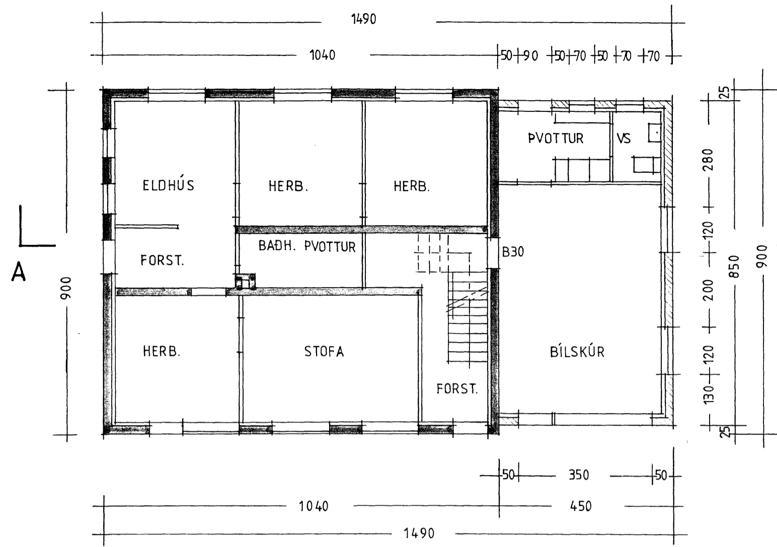
GRUNNMYND NEDRI HÆÐAR 1:100
