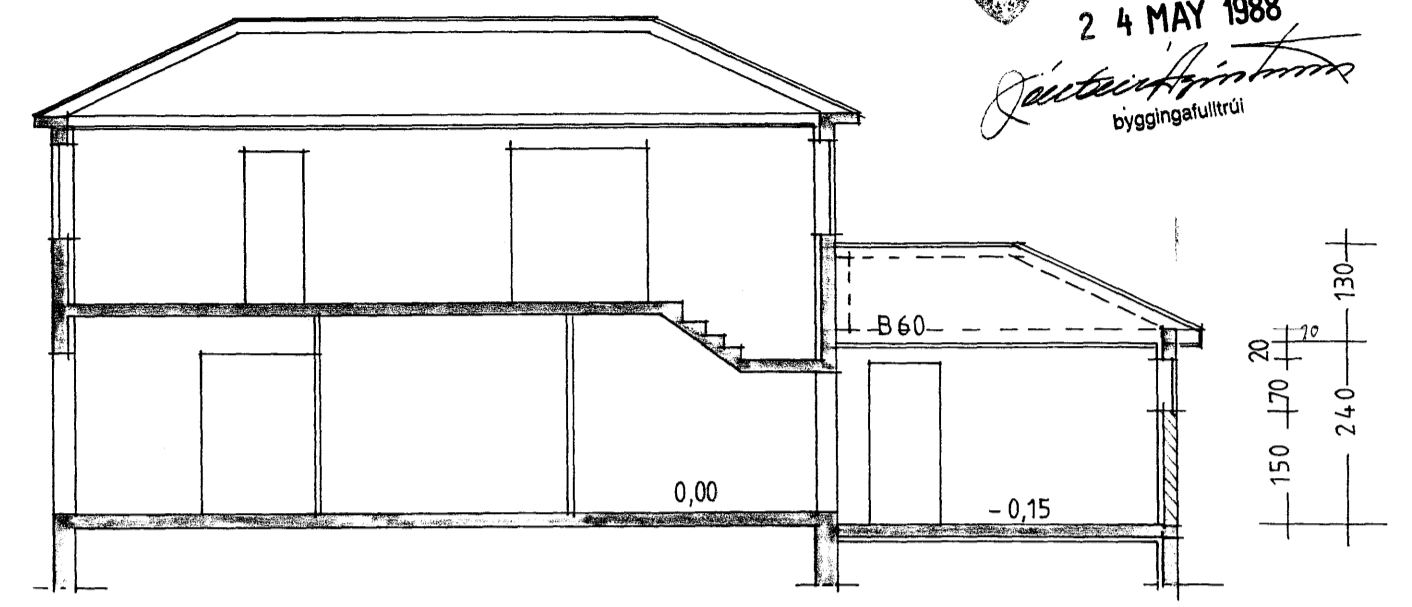
SNEIÐING A-A 1:100
