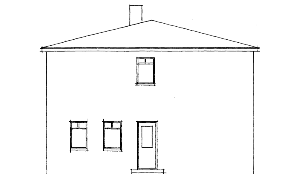
AUSTUR 1:100
